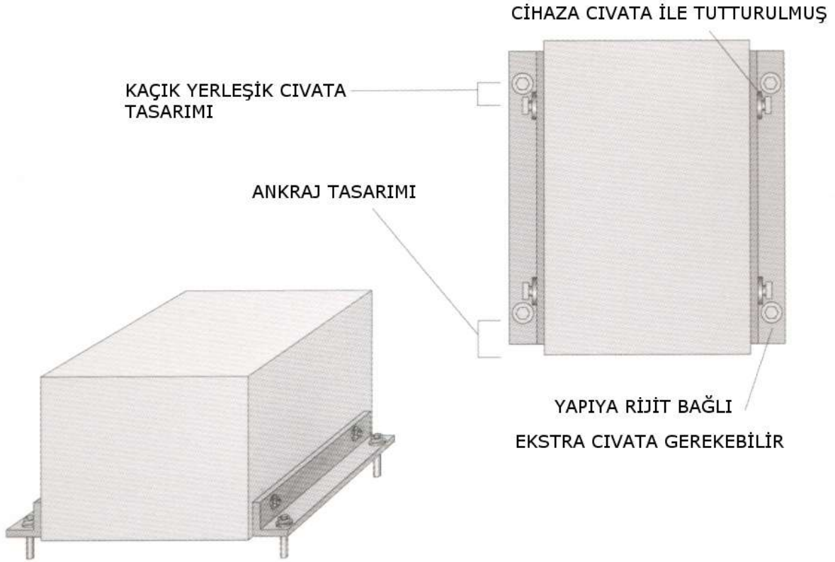
Şekil-3 Donanımın ileve takviye ile döşemeye sabitlenmesi*
